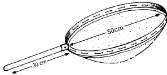
Sweep net
